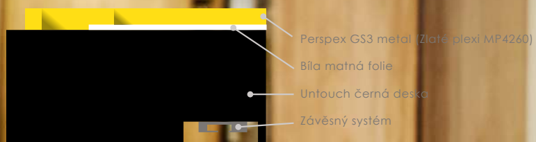
Orientační systém - destičky se jmenovkami na dveře kanceláří
